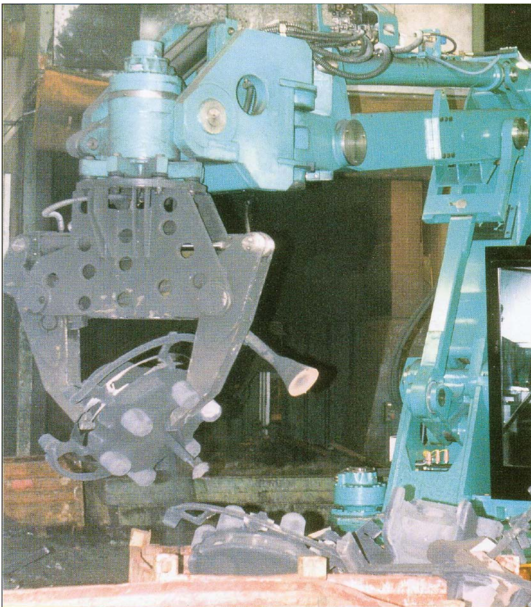
Манипулятор Clansman Dynamics C3010
