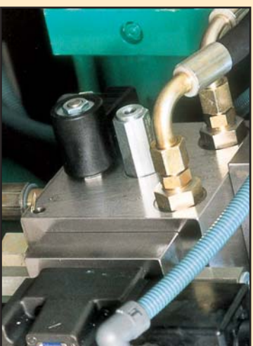
所有轴上都装有释放阀并在3个主轴上装有选择性压力限制装置
