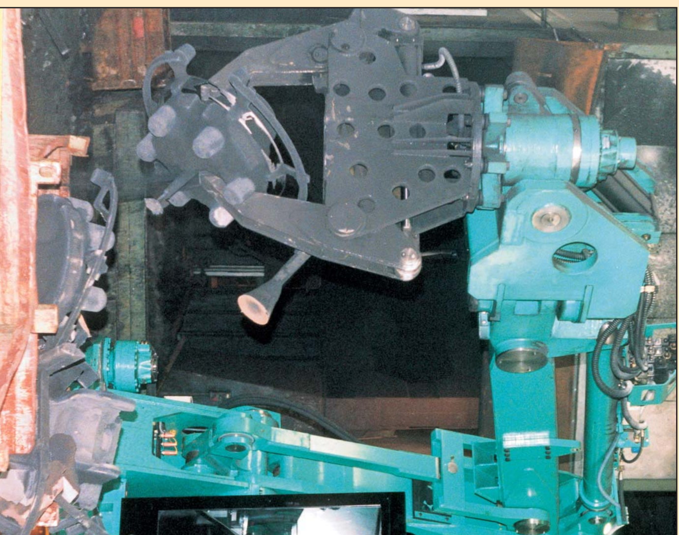
英国克莱斯曼C3010机械手
