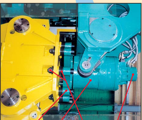
密封更换方便
